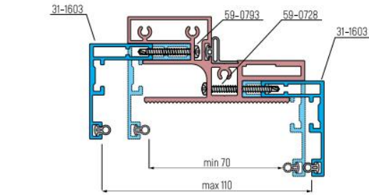
ADJUSTABLE DOOR FRAME - RANGES
