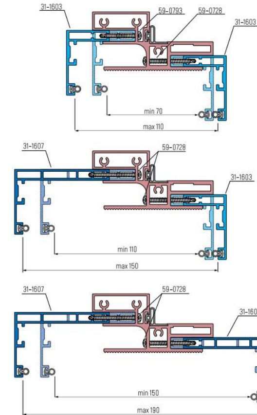
ADJUSTABLE DOOR FRAME - RANGES
